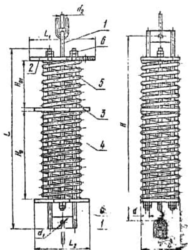
1 — тросер с тягами; 2 — основание верхнее; 3 — основание; 4 — пружина; 5 — пружина; 6 — гайка
